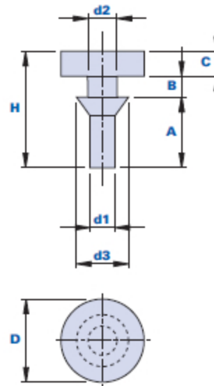
Abmessungen
